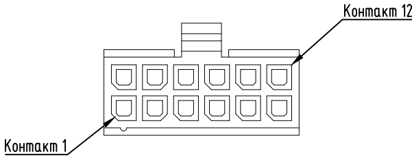
Рисунок 1 (масштаб 2:1)
